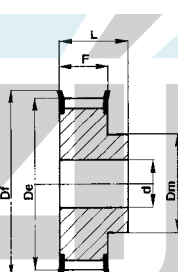
Tipo / Type 6F
