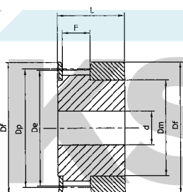
Tipo / Type 1F
